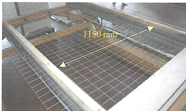
Fig. 4 – Assetto sperimentale campione B
