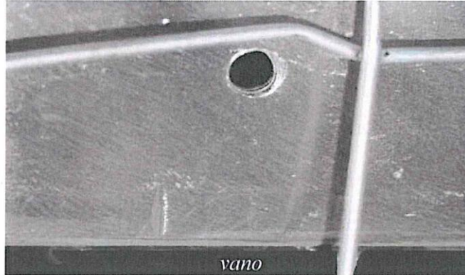
Fig. 13 – Campione A: dettaglio deformazione maglia della rete in prossimità punto di fissaggio centrale di destra
