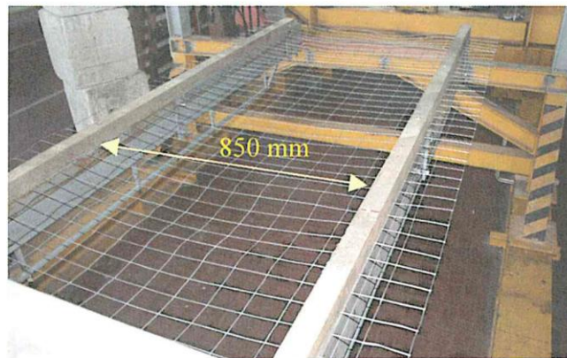
Fig. 2 – Assetto sperimentale campione A
