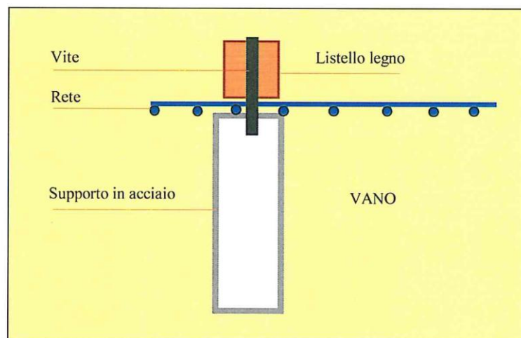
Fig. 1: Sezione schema di posa delle reti “First” sottoposte a prova
